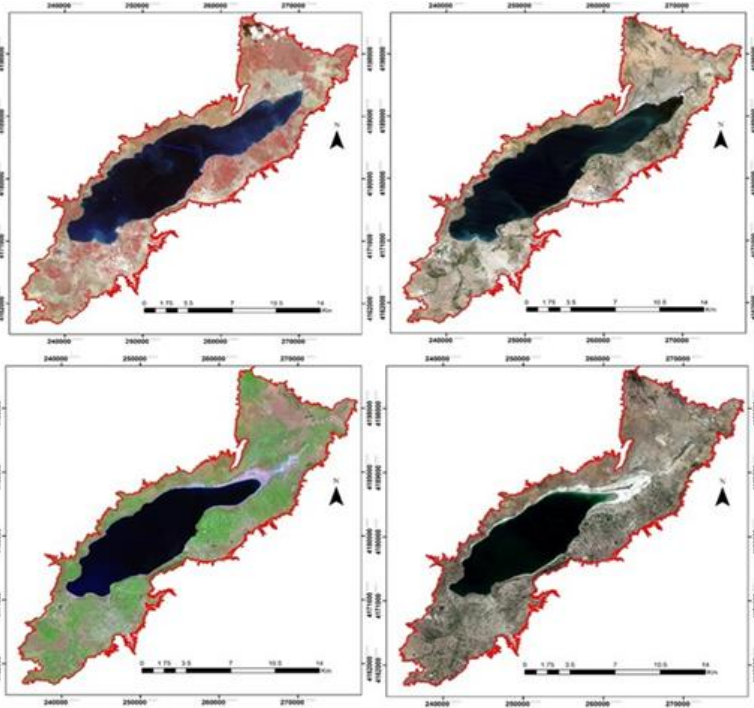
Fig 4. Satallite images of 1975 (a), 1987 (b), 2002 (c), 2017 (d) (Gözükara 2019).
